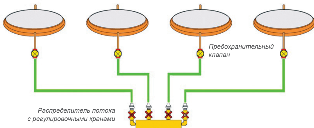
Диафрагменные домкраты
