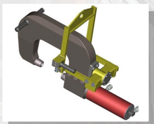
Гидравлическая скоба для клепки Кс25/200/95Г
